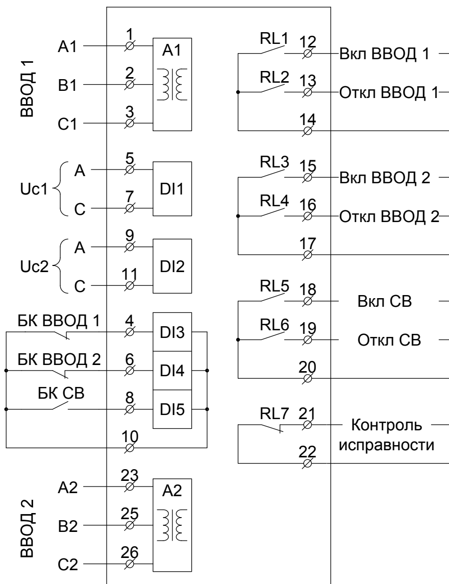
Схема подключения устройства СХ200.
