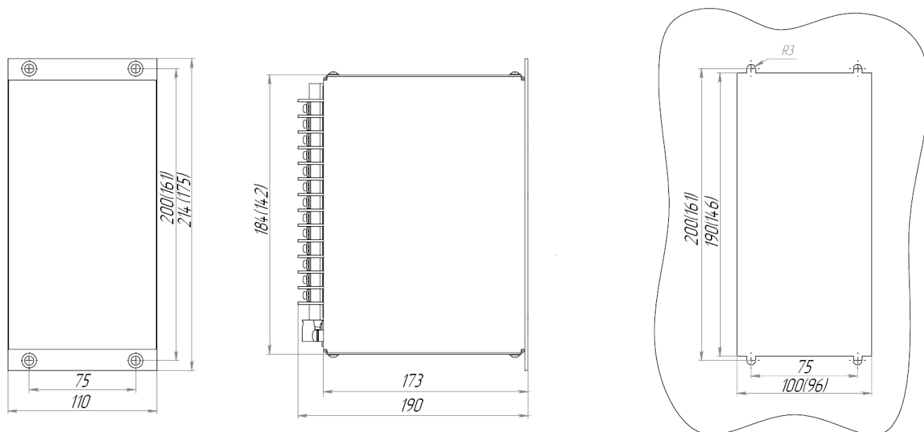
Габаритные и установочные размеры LX125, LX125k (В скобках для LX125k).
