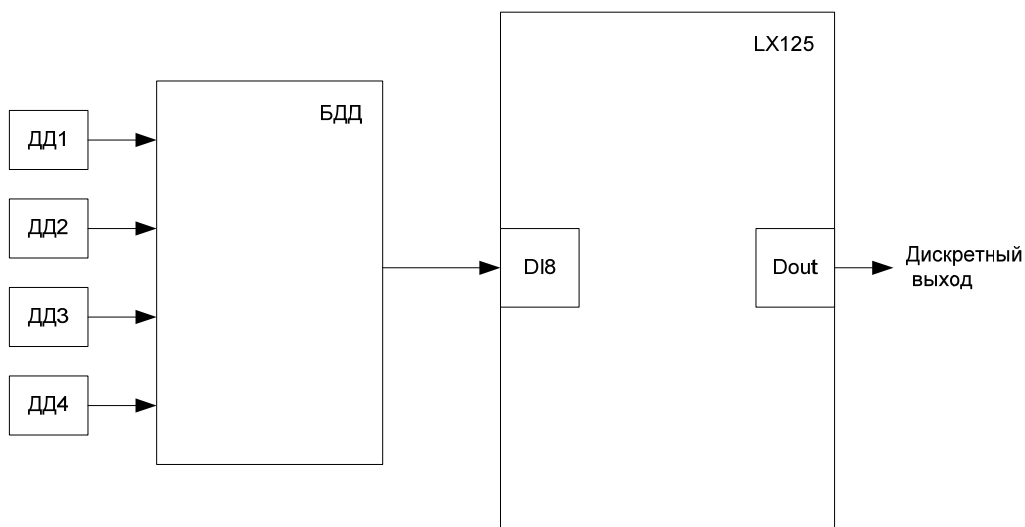
Рисунок 1. Структурная схема работы ДЗ.
