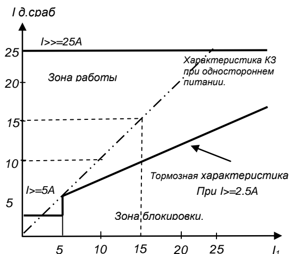
Рис.1. Тормозная характеристика дифзащиты с I \geq 2.5A и дифотсечка с I \geq 25A .
