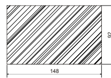
ВЫРЕЗАЕМОЕ ОТВЕРСТИЕ В ДВЕРИ РЕЛЕЙНОГО ШКАФА
