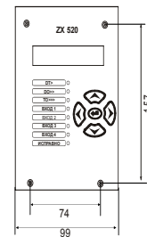
ВИД СПЕРЕДИ
