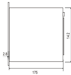
ВИД СБОКУ
