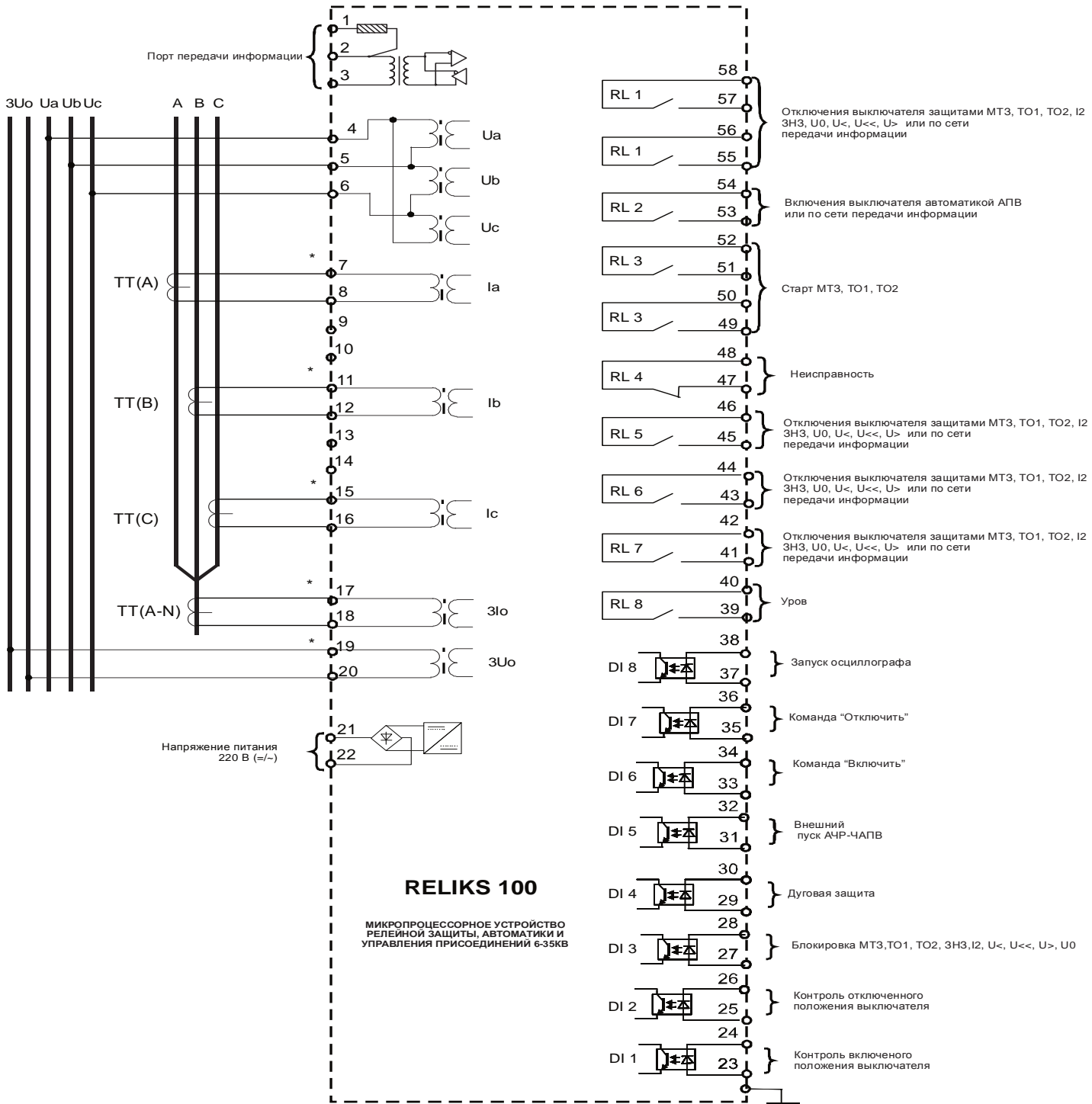
Схема подключения условная
